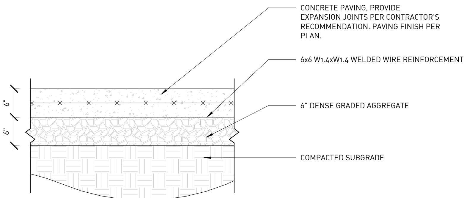
2 L401 'P2' CONCRETE PAVING SCALE: 1" = 1'-0"
