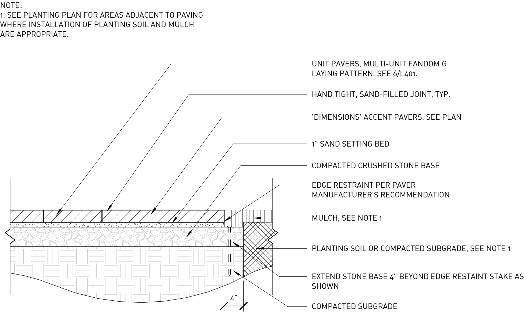
3 L401 'P3' UNIT PAVERS SCALE: 1" = 1'-0"
