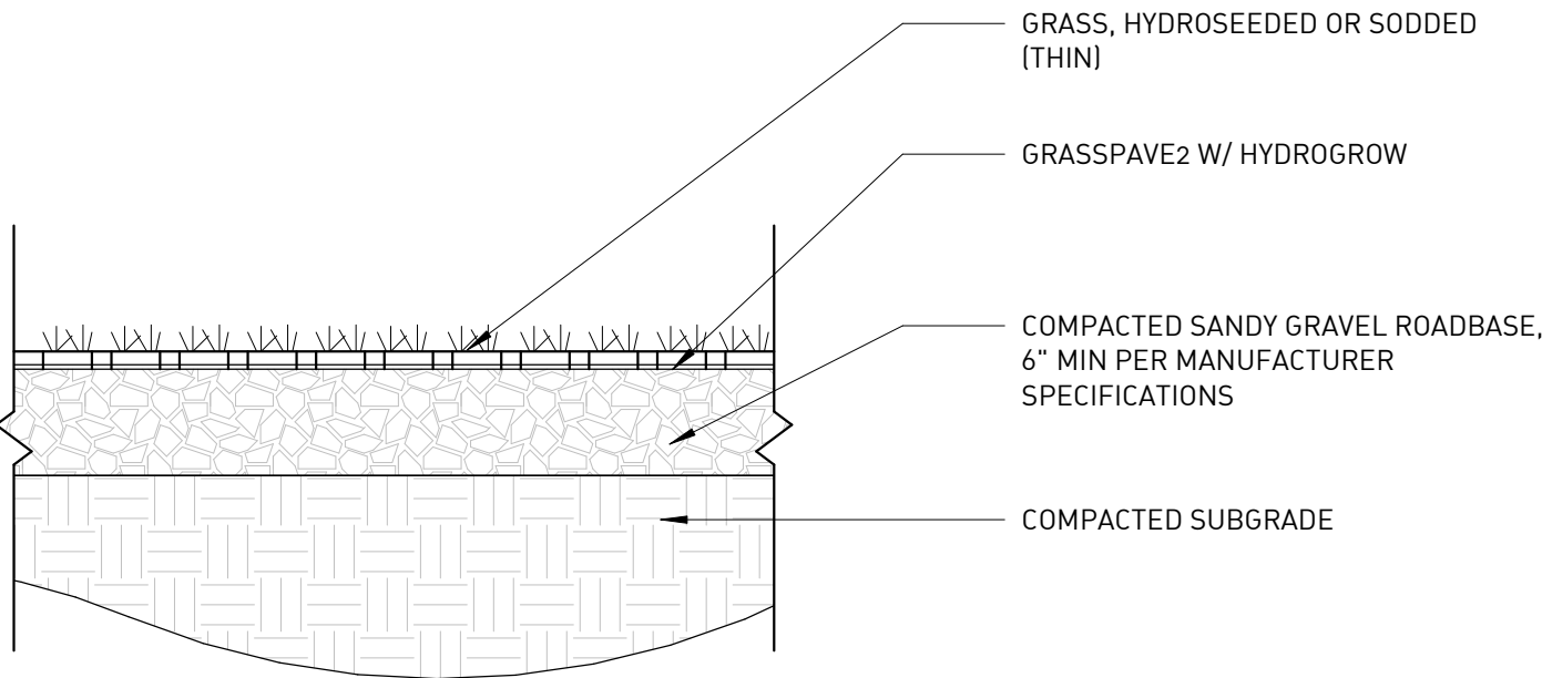
5 L401 'P4' GRASS PAVERS SCALE: 1" = 1'-0"
