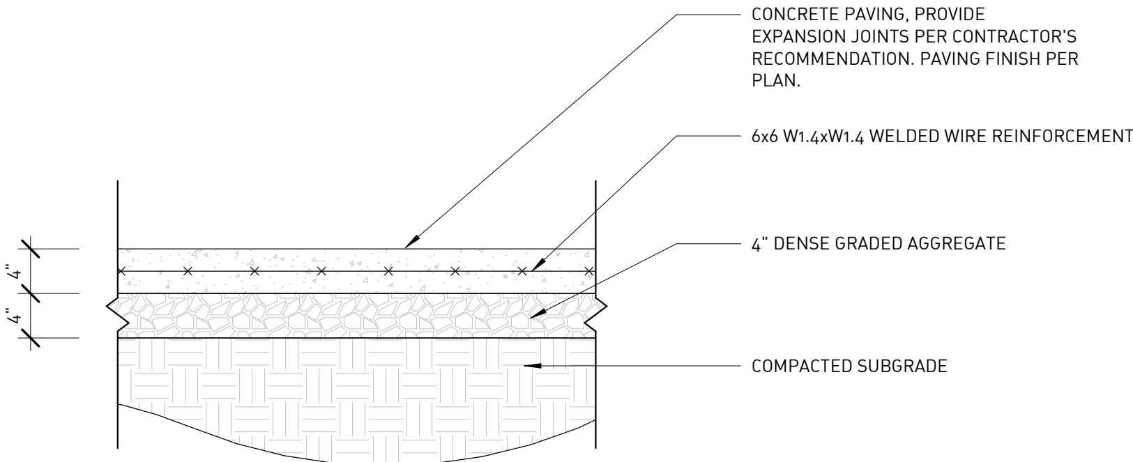
1 L401 'P1' CONCRETE PAVING SCALE: 1" = 1'-0"
