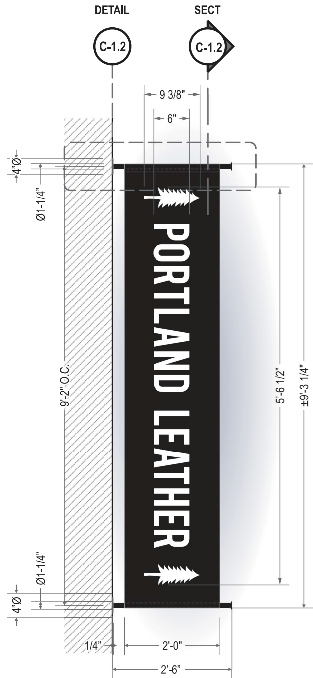
RIGHT SIDE SCALE: 1/2"=1'-0"
